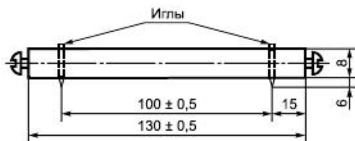
Рисунок 5 - Схема разметочного шаблона
