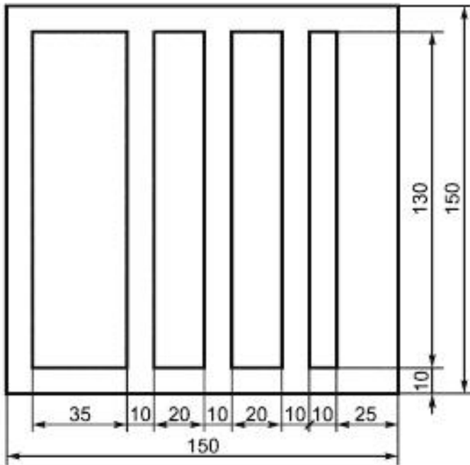
Рисунок 6 - Приспособление для разметки образца
