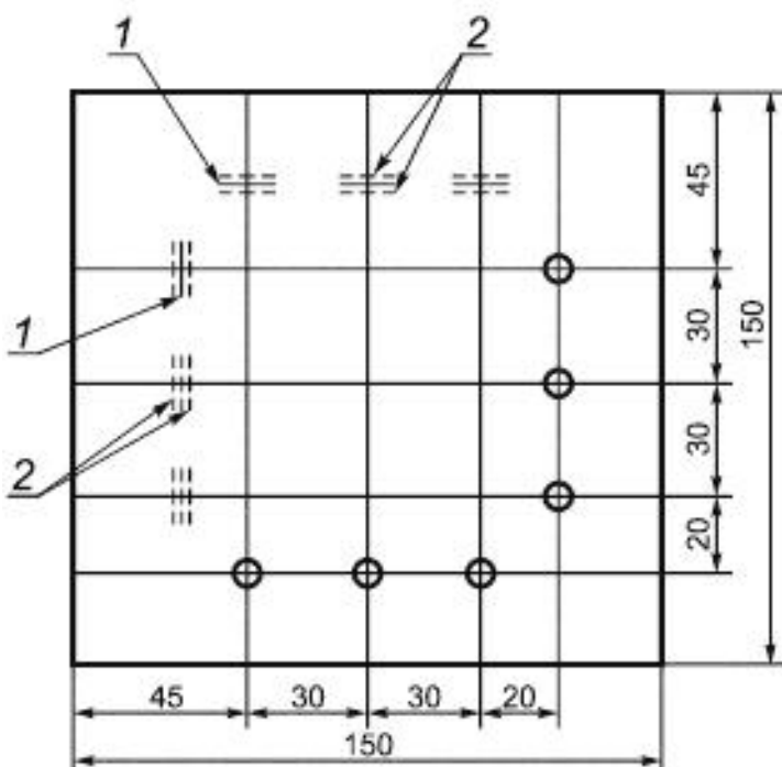
Рисунок 7 - Схема разметки образца
